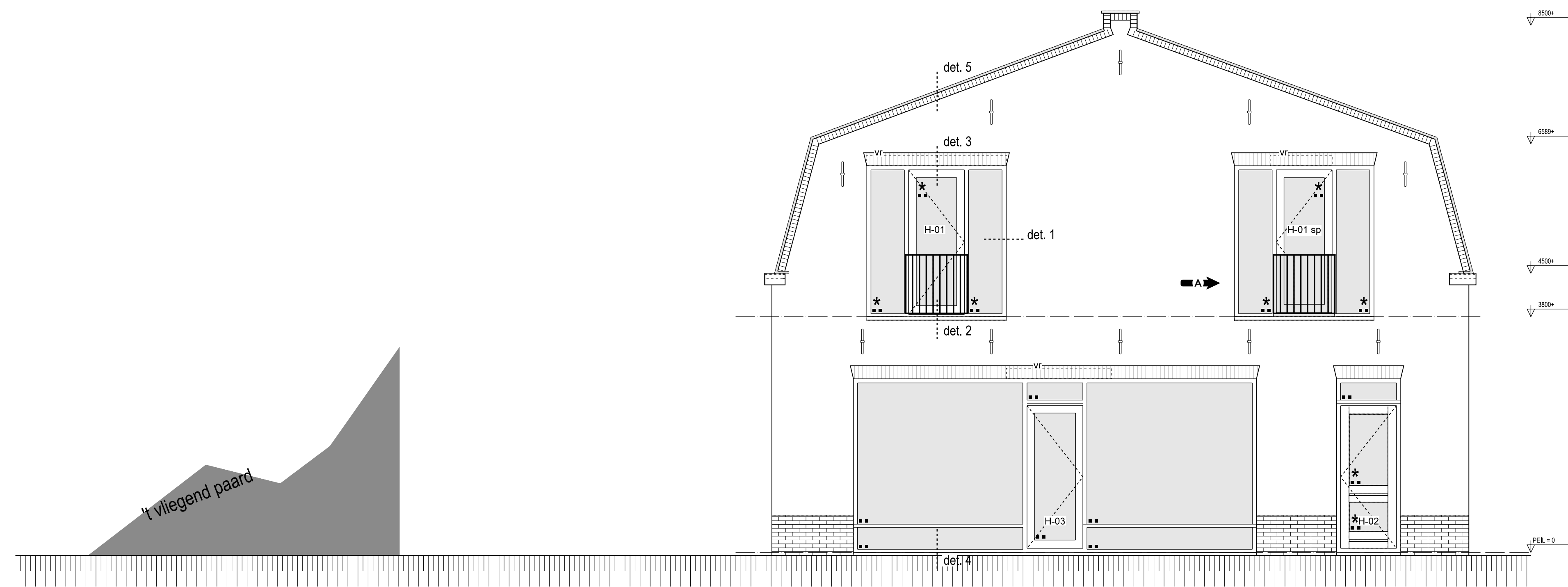
Voorgevel
