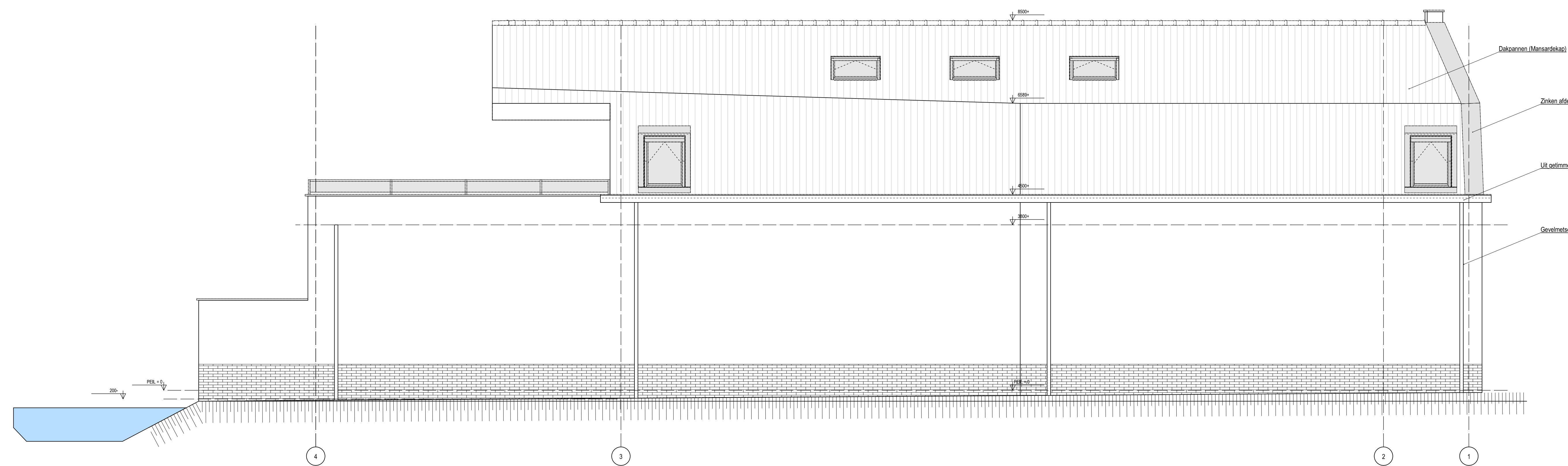
Linker zijgevel
