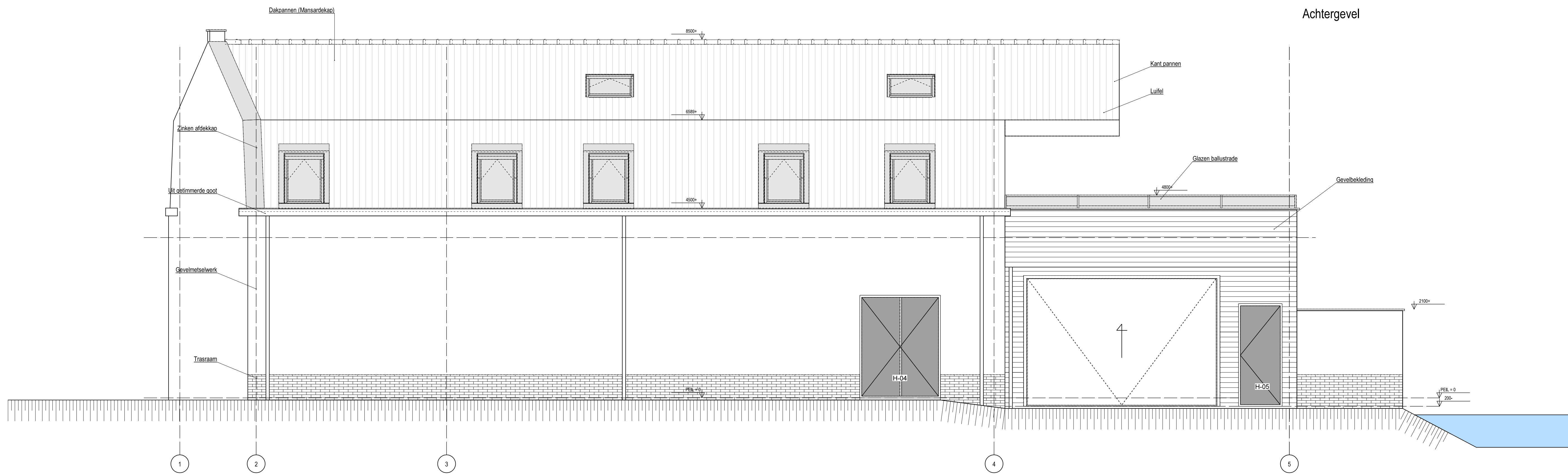
Rechter zijgevel
