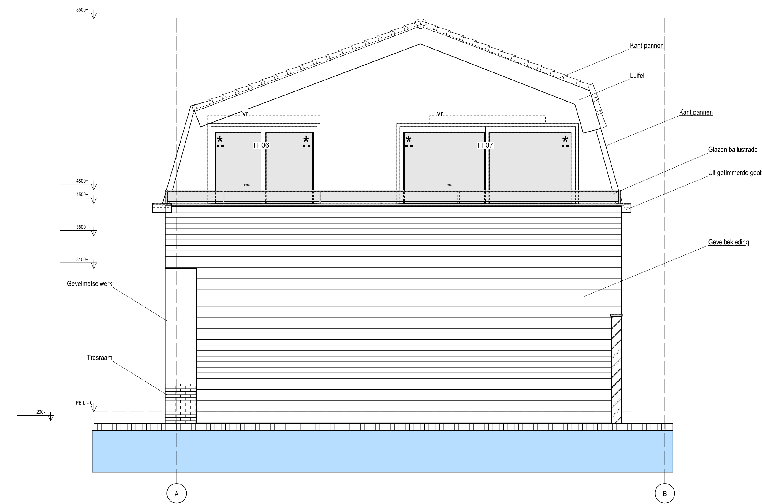
Achtergevel
